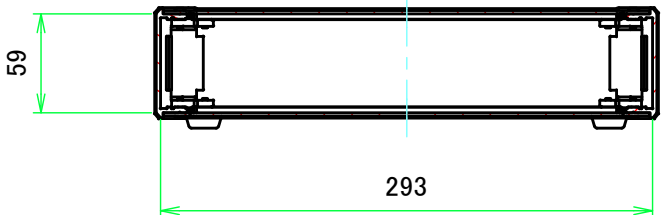
B-B ( 1:4.5 )
