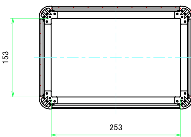
C-C ( 1:4.5 )
