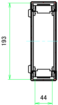
A-A ( 1:4.5 )
