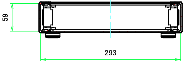
B-B ( 1:4.5 )
