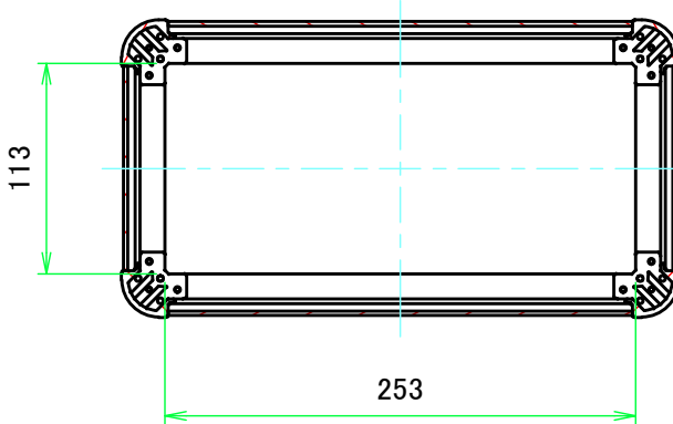
C-C ( 1:4.5 )
