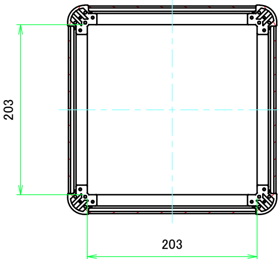
C-C ( 1:4.5 )
