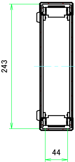
A-A ( 1:4.5 )
