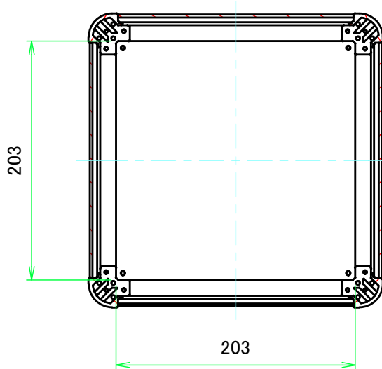
C-C ( 1:4.5 )
