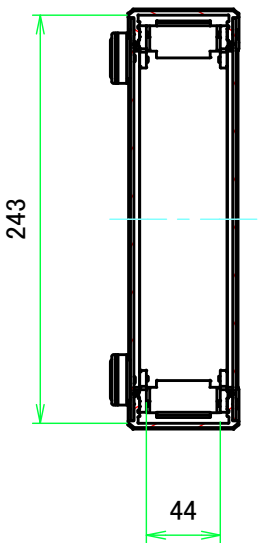
A-A ( 1:4.5 )
