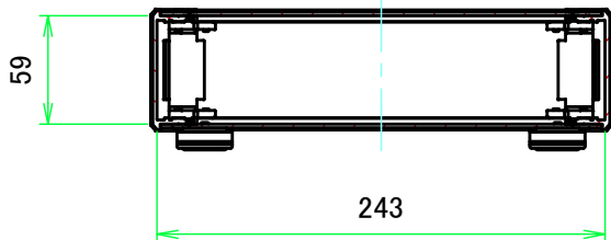
B-B ( 1:4.5 )
