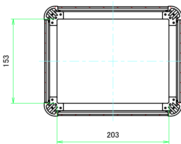
C-C ( 1:4 )
