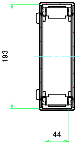
A-A ( 1:4 )
