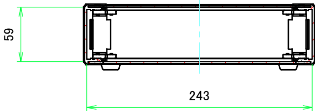
B-B ( 1:4 )
