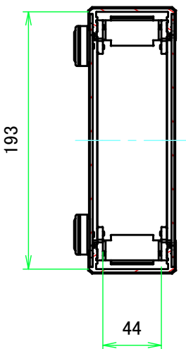
A-A ( 1:4 )
