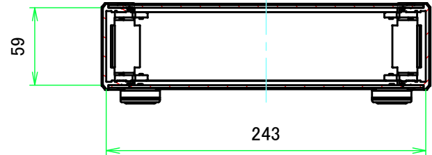
B-B ( 1:4 )
