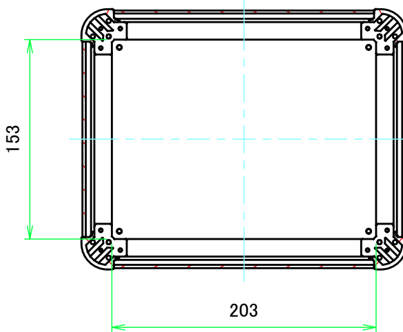
C-C ( 1:4 )
