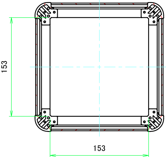
C-C ( 1:3.5 )
