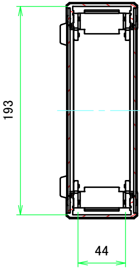
A-A ( 1:3.5 )
