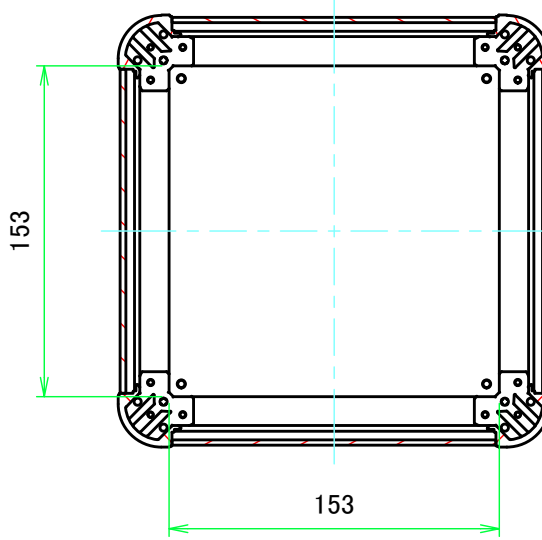
C-C ( 1:3.5 )
