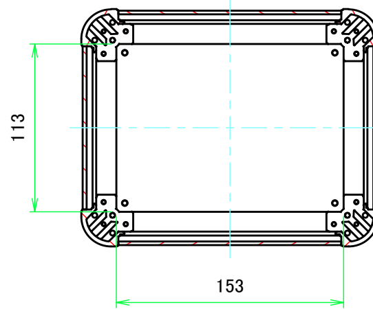
C-C ( 1:3.5 )
