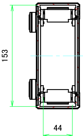
A-A ( 1:3.5 )
