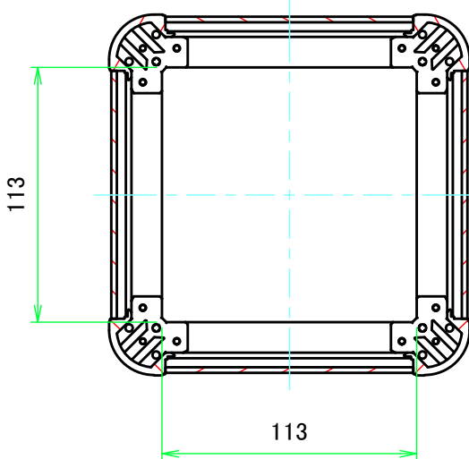
C-C ( 1:3 )
