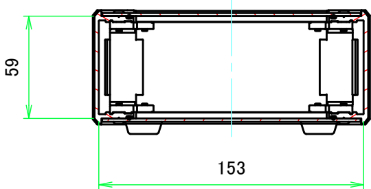
B-B ( 1:3 )
