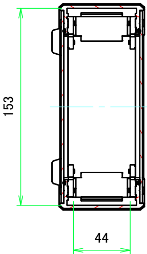
A-A ( 1:3 )
