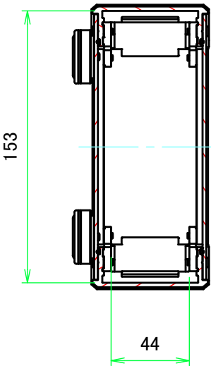
A-A ( 1:3 )
