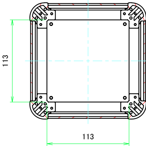
C-C ( 1:3 )
