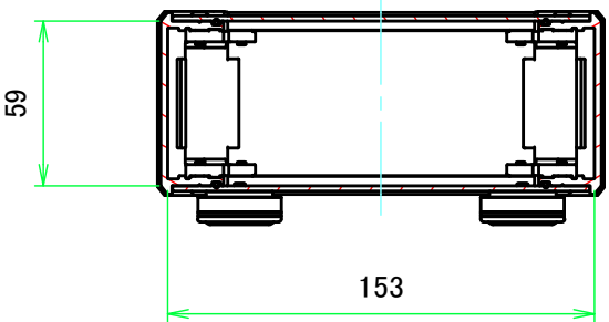
B-B ( 1:3 )
