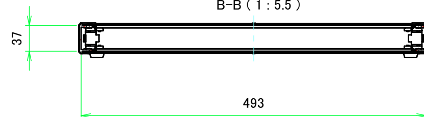
B-B (1 : 5.5)
