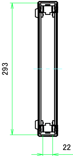
A-A (1:5)
