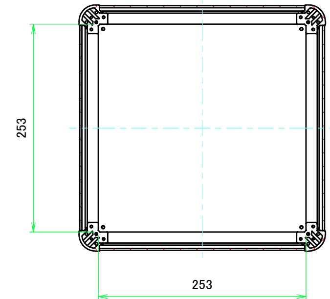
C-C ( 1 : 4.5 )
