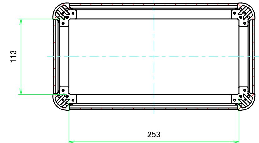
C-C (1:3.5)
