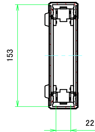
A-A (1:3.5)
