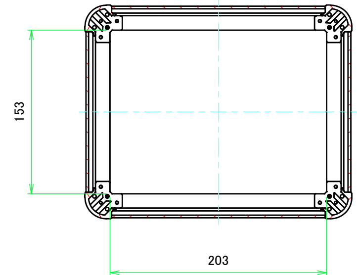
C-C ( 1 : 3.5 )
