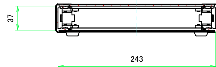
B-B ( 1 : 3.5 )
