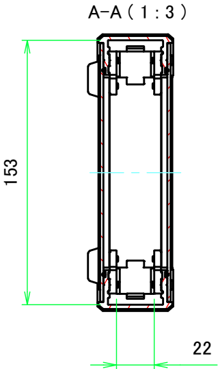
A-A (1:3)
