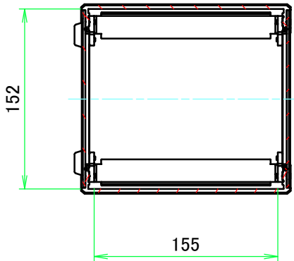
A-A ( 1 :4.5 )
