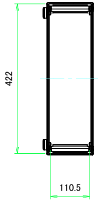
A-A (1:7.5)
