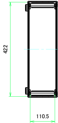
A-A (1:7)
