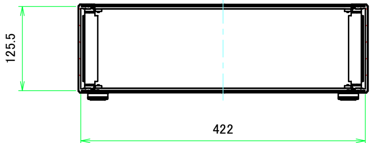
B-B ( 1 : 5.5 )
