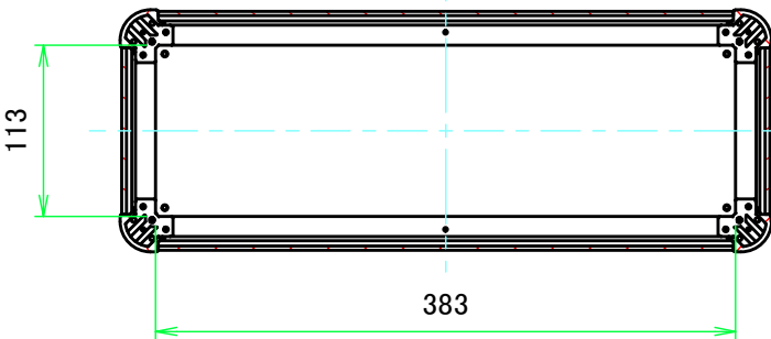
C-C ( 1 : 5.5 )
