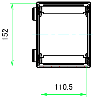
A-A ( 1 : 5.5 )
