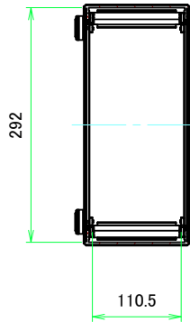
A-A (1:6)
