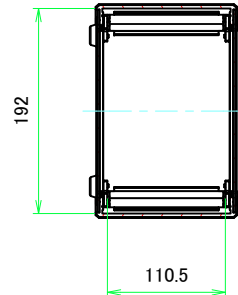
A-A (1:5)
