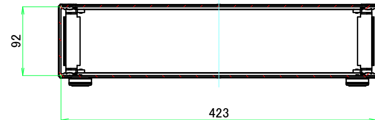
A-A (1:5)
