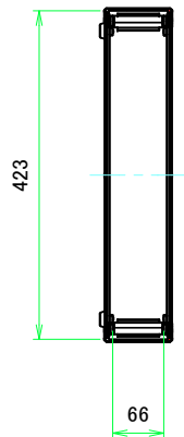
A-A (1:7.5)
