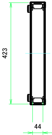
A-A ( 1:8 )
