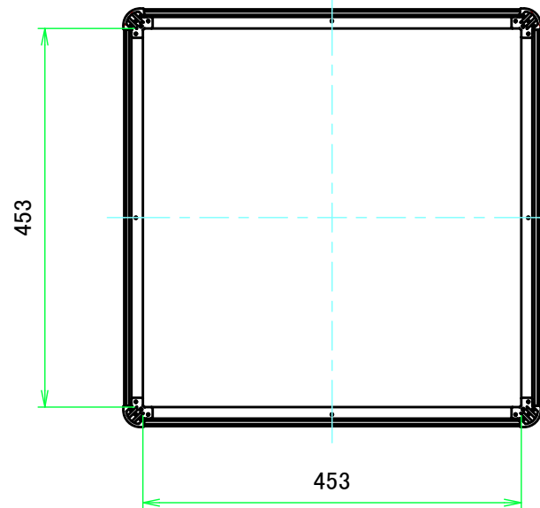
C-C ( 1:8 )
