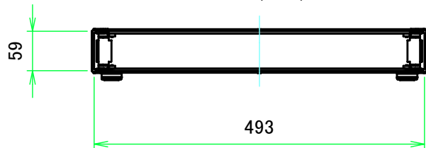
B-B ( 1:8 )
