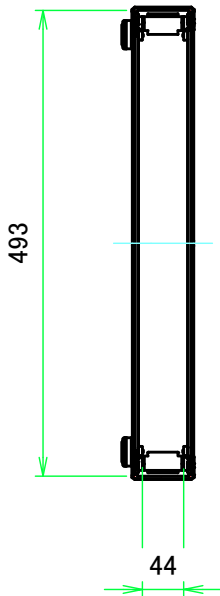
A-A ( 1:8 )
