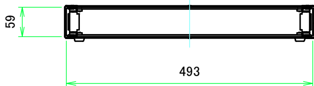
B-B ( 1:7.5 )
