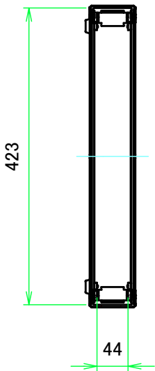
A-A ( 1:7.5 )
