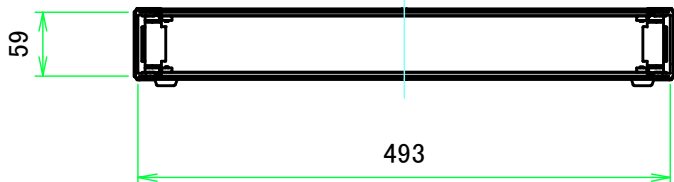
B-B ( 1:7 )
