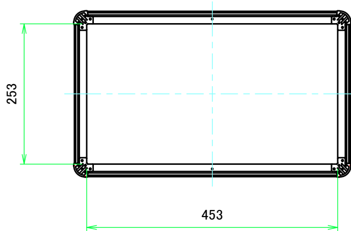
C-C ( 1:7 )
