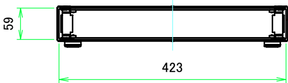
B-B ( 1:7 )
