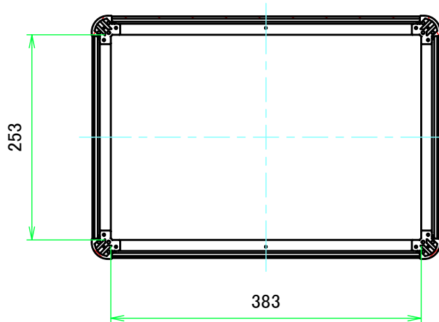
C-C ( 1:6.5 )
