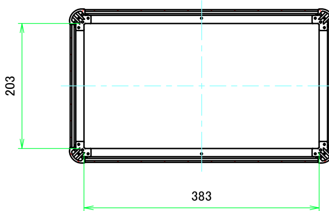
C-C ( 1:6 )
