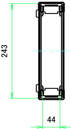
A-A ( 1:6 )
