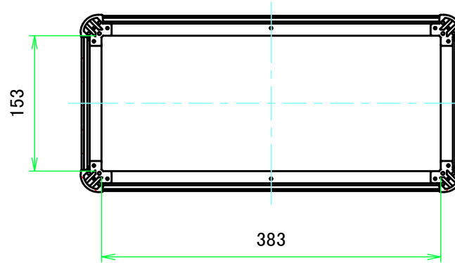
C-C ( 1:6 )
