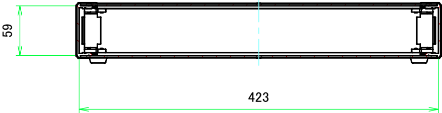
B-B ( 1 : 4.5 )
