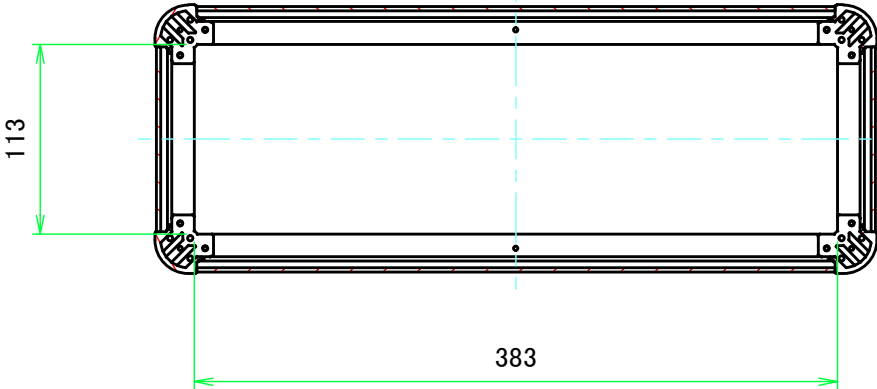
C-C ( 1 : 4.5 )
