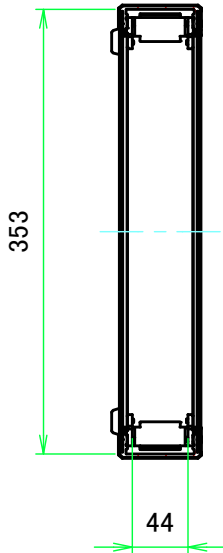
A-A ( 1:6 )
