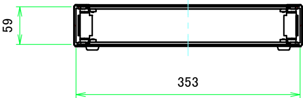
B-B ( 1:6 )
