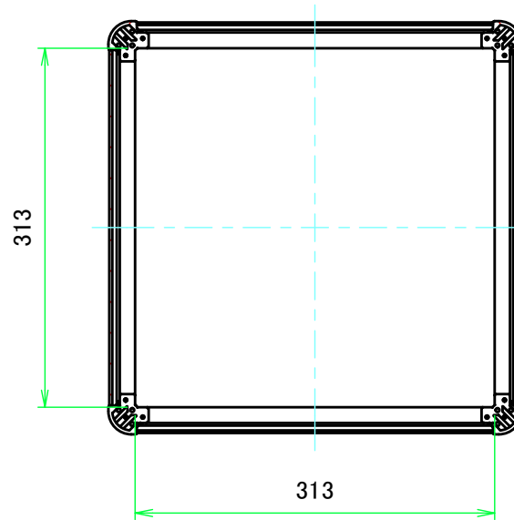
C-C ( 1:6 )
