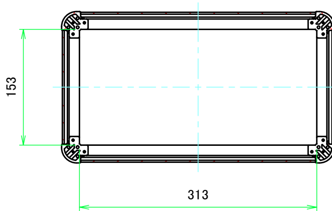
C-C ( 1:5 )
