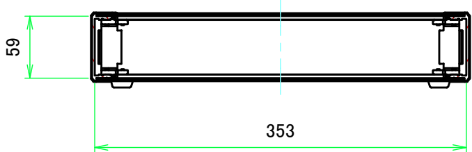
B-B ( 1:5 )
