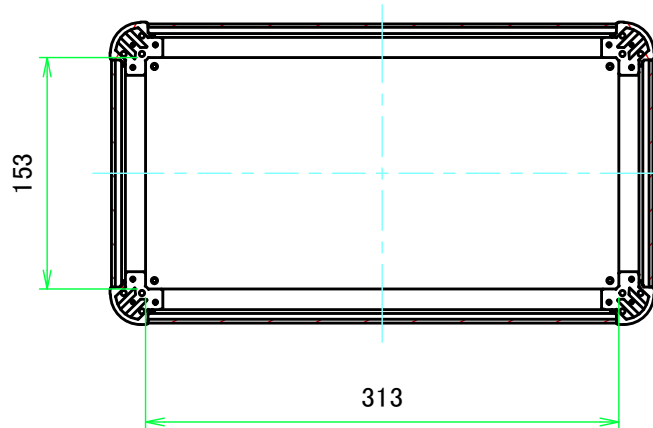
C-C ( 1:5 )
