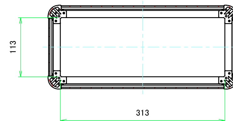
C-C (1 : 4.5)
