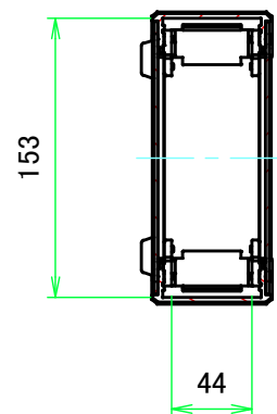
A-A (1 : 4.5)
