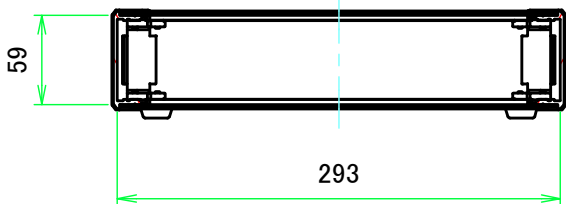
B-B ( 1:5 )
