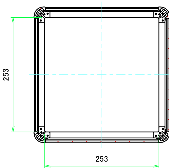
C-C ( 1:5 )
