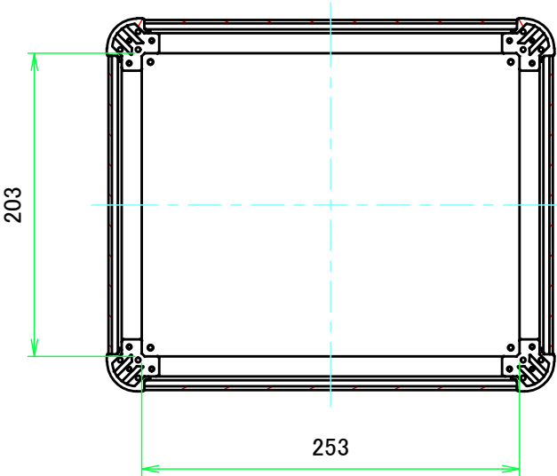
C-C ( 1:4.5 )
