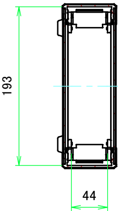
A-A ( 1:4.5 )
