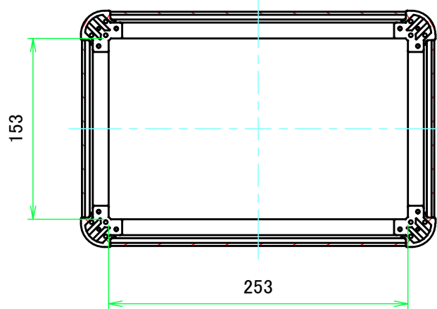
C-C ( 1:4.5 )
