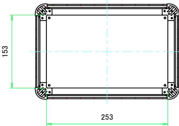
C-C ( 1:4.5 )
