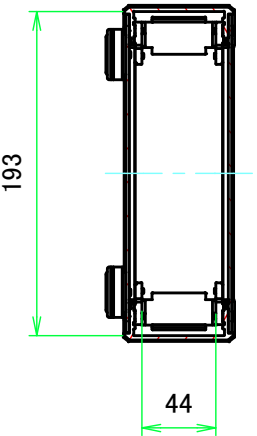
A-A ( 1:4.5 )
