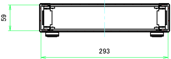
B-B ( 1:4.5 )
