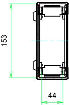
A-A ( 1:4.5 )
