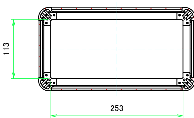
C-C ( 1:4.5 )
