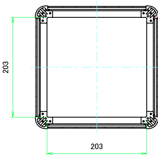
C-C ( 1:4.5 )
