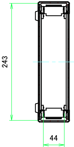
A-A ( 1:4.5 )
