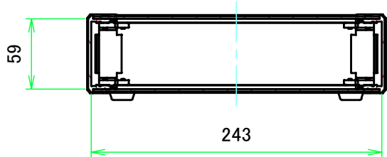
B-B ( 1:4.5 )
