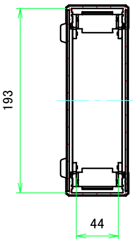
A-A ( 1:4 )
