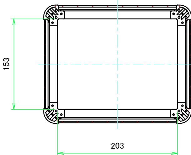
C-C ( 1:4 )
