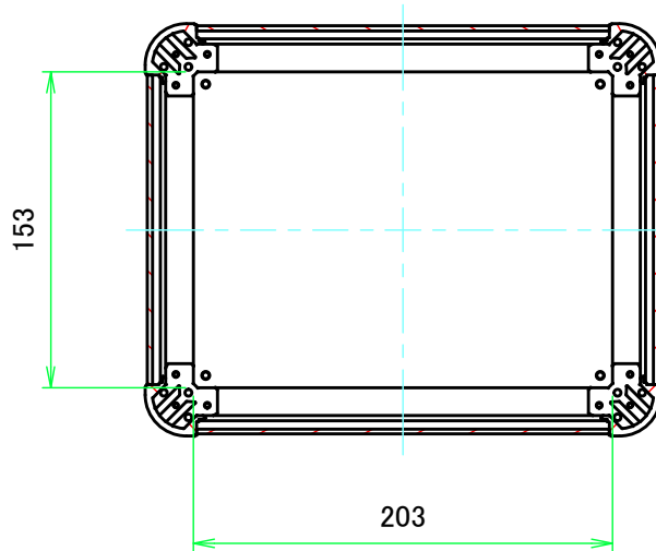
C-C ( 1:4 )
