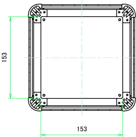
C-C ( 1:3.5 )
