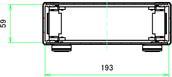
B-B ( 1:3.5 )
