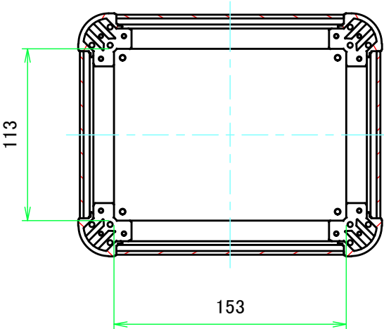
C-C ( 1:3.5 )
