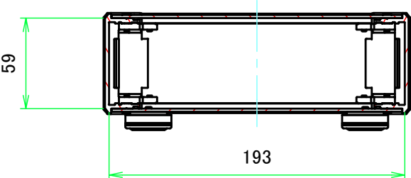
B-B ( 1:3.5 )
